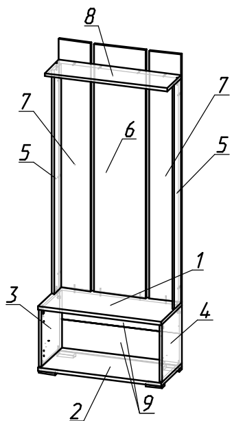
Рис.1 Схема сборки
